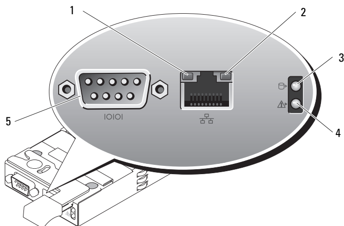
Figure 1-4. Caractéristiques du module DRAC/MC
